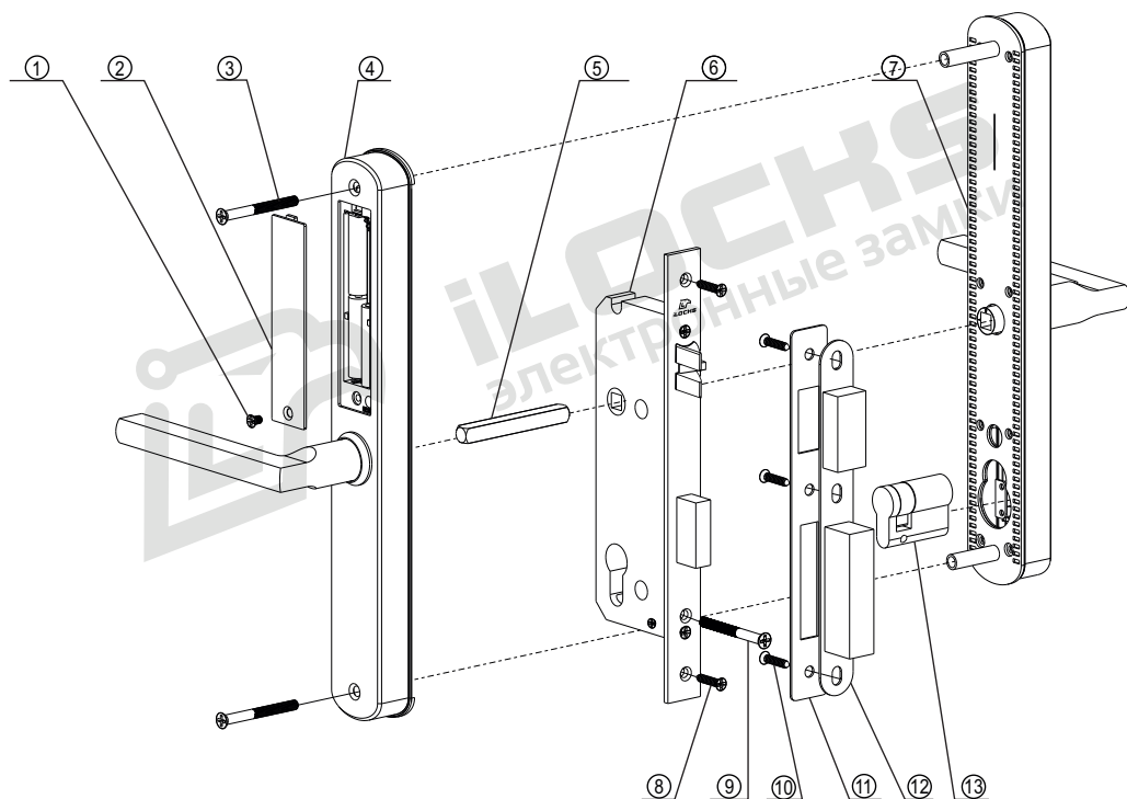
Рисунок №1 – Структурная схема (спецификация) замков типа iLOCKS IS210AB-BBL 433+BLE
