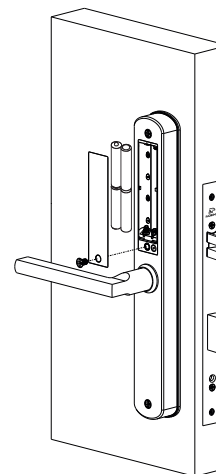
Рисунок №9 – Установка батарей типа AAA
