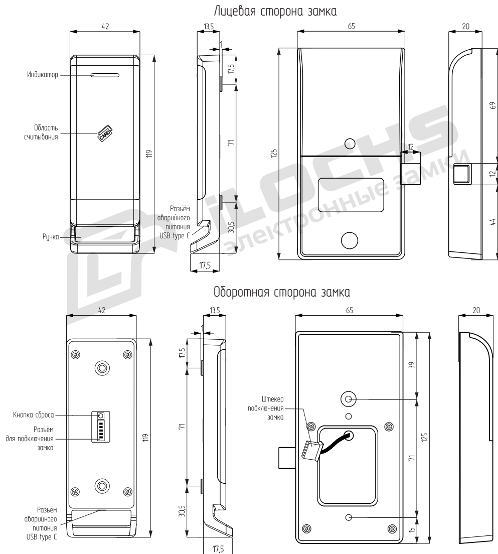
Рисунок №1 – Габаритные характеристики замка для шкафчиков IS0870-MF
