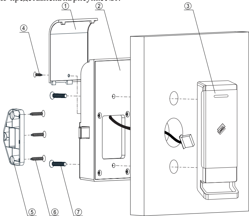
Рисунок №2 – Структурная схема (спецификация) замка IS0870-MF
