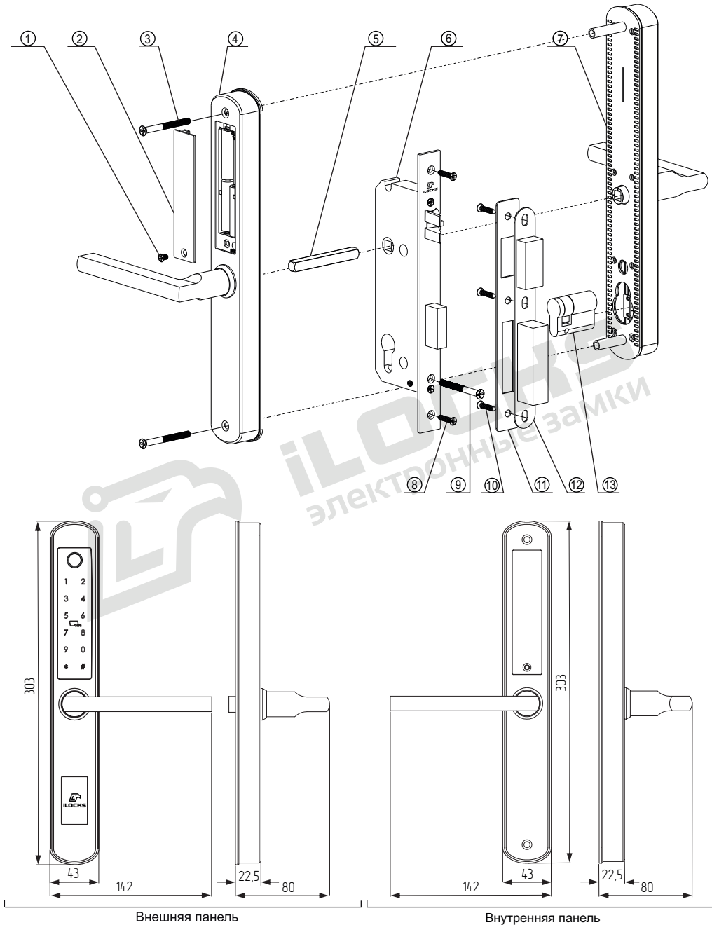
Рисунок №1 – Структурная схема (спецификация) и габариты замков типа iLOCKS IS210AB-BBL 433+BLE
