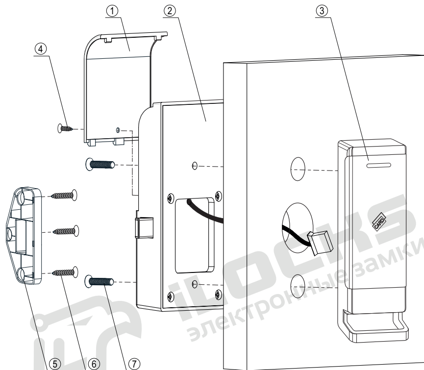
Рисунок №1 – Структурная схема (спецификация) электронного замка для шкафчиков IS0870-MF
