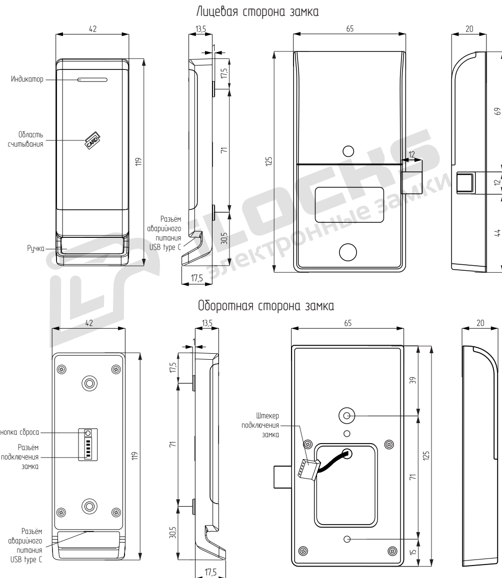
Рисунок №2 – Габаритные характеристики электронного замка IS0870-MF
